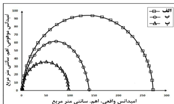
شکل ۷- نمودار نایکویست مربوط به آزمایش طیف سنجی امپدانس الکتروشیمیایی در حداقل سه بار تکرارپذیری: الف) فلز پایه، ب) فلز جوش ایجاد شده با حرارت ورودی ۶/۷۵ kJ/mm، پ) فلز جوش ایجاد شده با حرارت ورودی ۱۱/۲۵ kJ/mm
