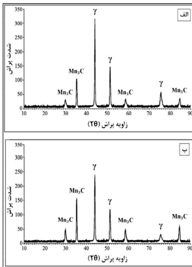
شکل ۵- الگوهای XRD از فلز جوش اتصال جوشکاری ایجاد شده با حرارت ورودی: الف) ۶/۷۵ kJ/mm، ب) ۱۱/۲۵ kJ/mm
