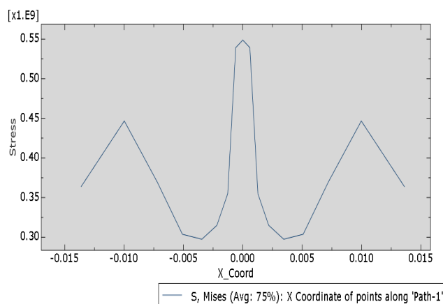
شکل ۱۲ - تنشهای پسماند روی سطح فلز در مقطع عرضی
