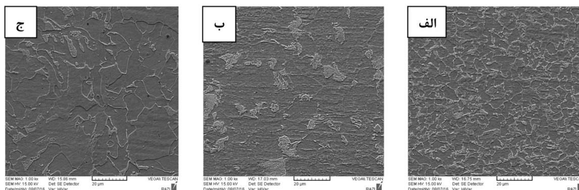
شکل 6-الف) تصاویر میکروسکوپی ناحیه متأثر از حرارت، ب) ریشه جوش و ج) منطقه جوش در موقعیت 7/30-6
