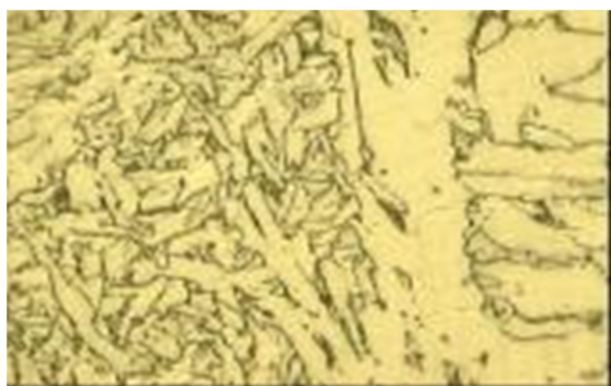
شکل 12- تصاویر میکروسکوپی پاس ریشه
