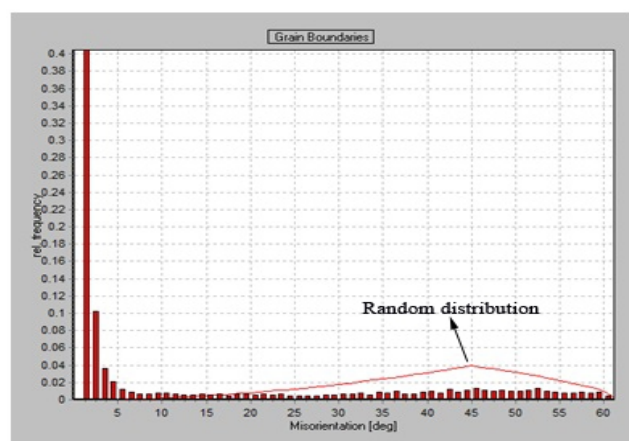
شکل 8- توزیع مرزانه های نانوکامپوزیت \text{Al-4n6mAl}_2\text{O}_3 جوشکاری شده با (الف) سرعت 1900rpm و سرعت خطی 37mm/min (ب) سرعت 2000 rpm و سرعت خطی 40mm/min
