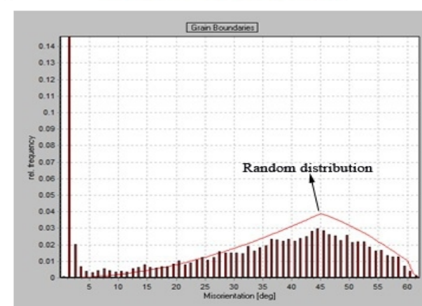
شکل 7- توزیع مرزانه های نانوکامپوزیت \text{Al-4n6mAl}_2\text{O}_3 جوشکاری شده با (الف) سرعت 1600rpm و سرعت خطی 32mm/min (ب) سرعت 1600rpm و سرعت خطی 40mm/min
