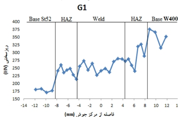
شکل ۱۰- تغییرات ریزسختی در جوش، منطقه متأثر از حرارت و فلز پایه نمونه G1.
