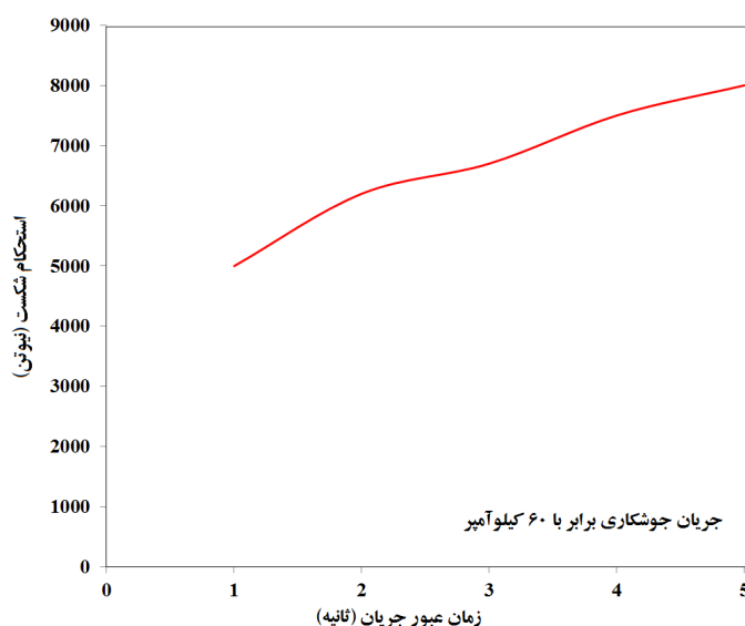
شکل 10- تغییرات استحکام شکست نمونه های جوشکاری شده با جریانی برابر با 60 کیلوآمپر و زمان های مختلف عبور جریان از الکتروودها.
