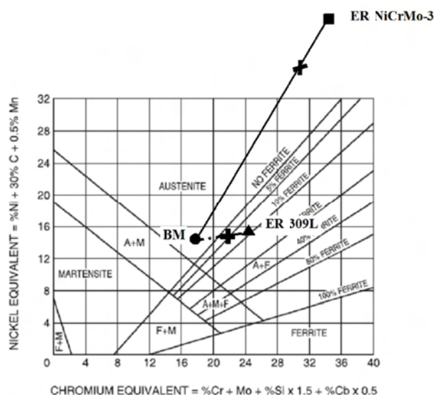
شکل 1- پیش‌بینی ساختار فلزپایه و فلزپرکننده \gamma ، \delta ، \gamma + \delta به ترتیب معرفی فلزجوش حاصل از ER309L و ERNiCrMo-3.
