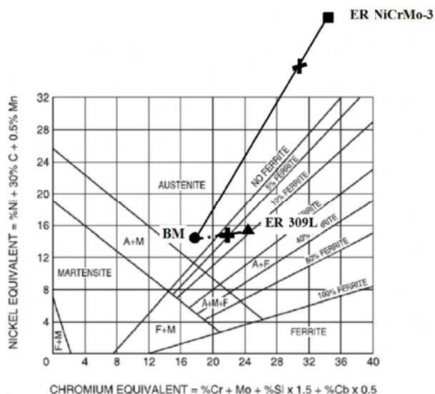
شکل 1- پیش‌بینی ساختار فلزپایه و فلزپرکننده. \times ، \bullet به ترتیب معرفی فلزجوش حاصل از ERNiCrMo-3 و ER309L
