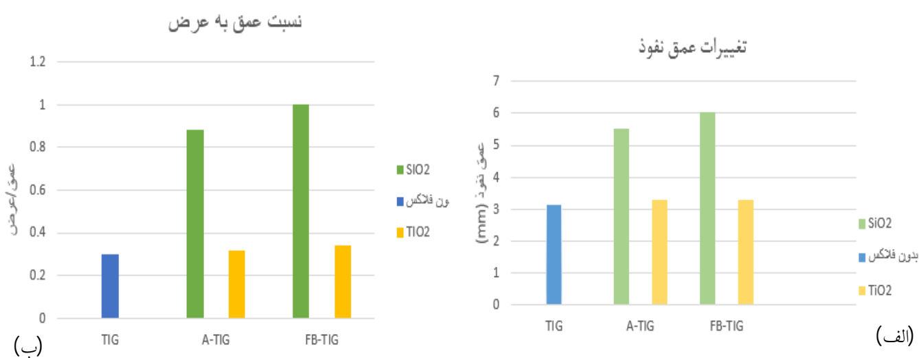
شکل 4- نمودارهای مقایسه عمق نفوذ و (ب) نسبت عمق به عرض نمونه‌های مرحله اول
