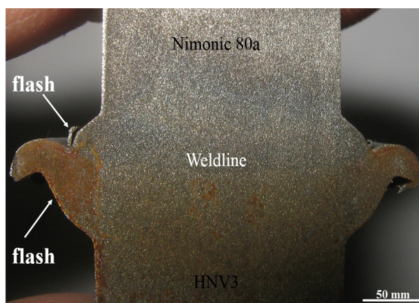
شکل ۱- سطح مقطع اتصال و فلش شکل گرفته در هر دو ناحیه فولادی و سوپراآلیاژی.
