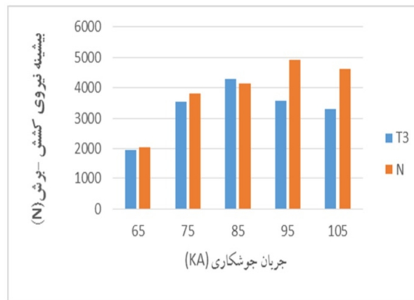
شکل 4- نمودار ستونی نیروی کشش برش بر حسب جریان جوشکاری برای نمونه های نانو ساختار و آلومینیوم تجاری T3-2024.
