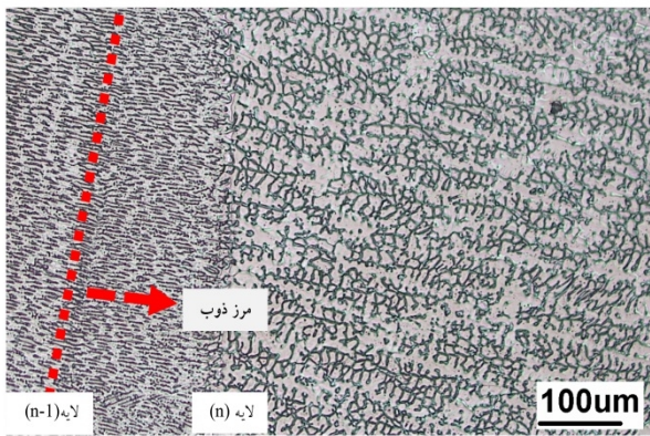
شکل 8- تصویر میکروسکپ نوری در امتداد مقطع عرضی در یک‌لایه، ریزساختار لایه‌ها و همچنین شاخصی را نشان می‌دهد که نشان می‌دهد حالت انجماد به تدریج از آستنیت ( \gamma ) اولیه و فریت ( \delta ) ثانویه (A/F) به فریت ( \delta ) اولیه و آستنیت ( \gamma ) ثانویه (F/A)، در یک‌لایه تغییر می‌کند
