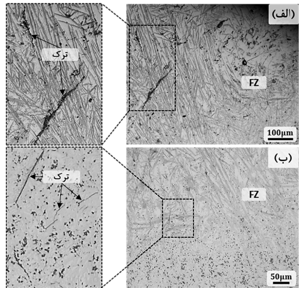
شکل 9- تصویر میکروسکوپی نوری از ترک‌های موجود در بخش فلز جوش چدن خاکستری جوشکاری شده به روش SMAW با الکتروود E6013.
