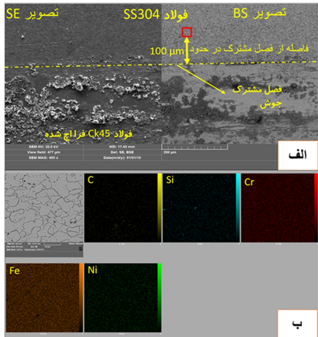
شکل 16- نتایج بررسی به کمک میکروسکوپ الکترونی برای نمونه B52 به همراه ریزساختار و آنالیز عنصری صفحه‌ای ناحیه‌ی جوش (مربع قرمز رنگ).
