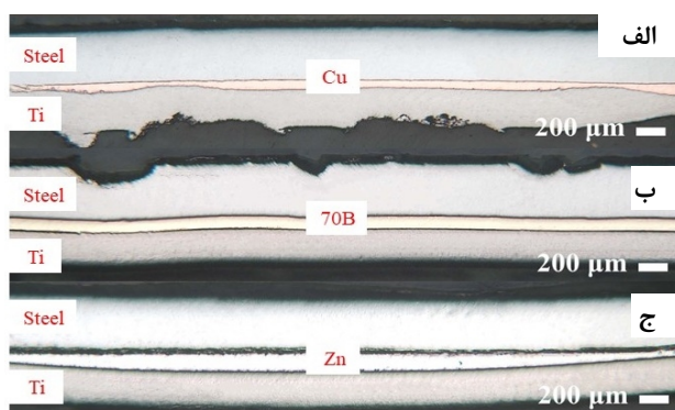
شکل 2- سطح مقطع نمونه‌های جوشکاری الف - با لایه میانی مس خالص، ب - با لایه میانی B70 و ج - با لایه میانی روی خالص قبل از اچ
