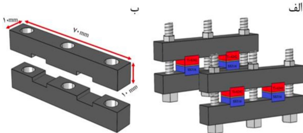
شکل 2- الف - نحوه استقرار اجزا اتصال در داخل نگهدارنده ب - طرح‌واره نگهدارنده اتصال ساخته شده.
