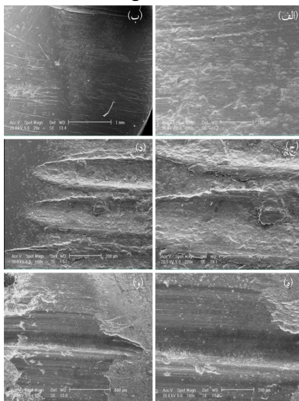
شکل 18- تصاویر SEM از سطح سایش روکش (Fe, Cr)_3Al در دماهای، الف و ب - 25°C، ج و د - 200°C و ه و ز - 500°C
