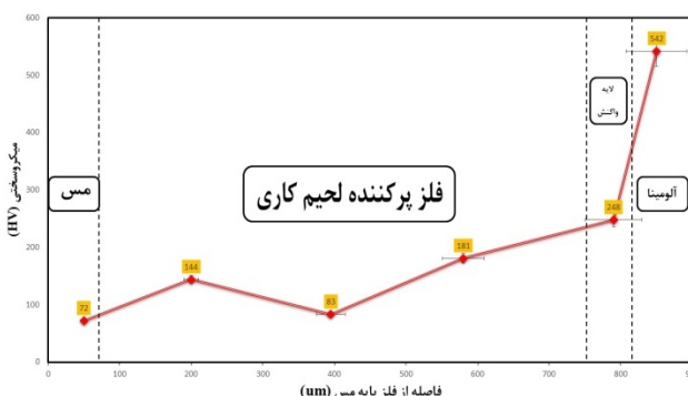
شکل 18- نمودار ریزسختی ویکرز اتصال آلومینا به مس با فلز پرکننده
