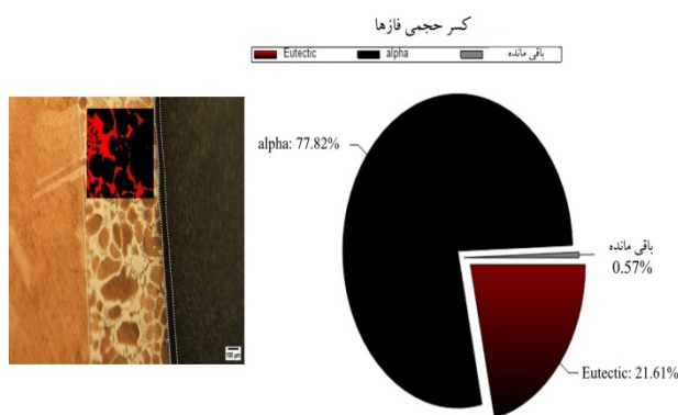
شکل 7- کسر حجمی فاز یوتکتیک و فاز اولیه \alpha اتصال با فلز پرکننده \text{Ag-Cu-Ti-Sn-3.5Zr} با استفاده از نرم افزار Mip.
