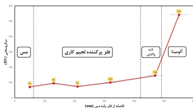
شکل 17- نمودار ریزسختی ویکرز اتصال آلومینا به مس با فلز پرکننده
