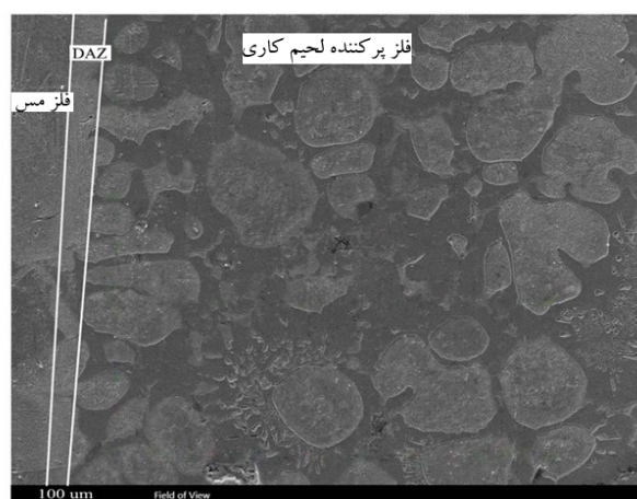
شکل 15- تصویر میکروسکوپی الکترونی روبشی از اتصال Al_2O_3/Cu با فلز پرکننده Ag-Cu-Ti-Sn-3.5Zr
