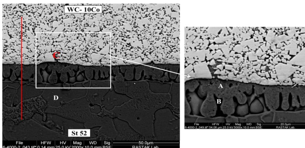
شکل 4- تصویر میکروسکوپ الکترونی روبشی از اتصال ایجاد شده در دمای 1100 درجه سانتی گراد و زمان نگهداری یک دقیقه با استفاده از لایه میانی مس.
