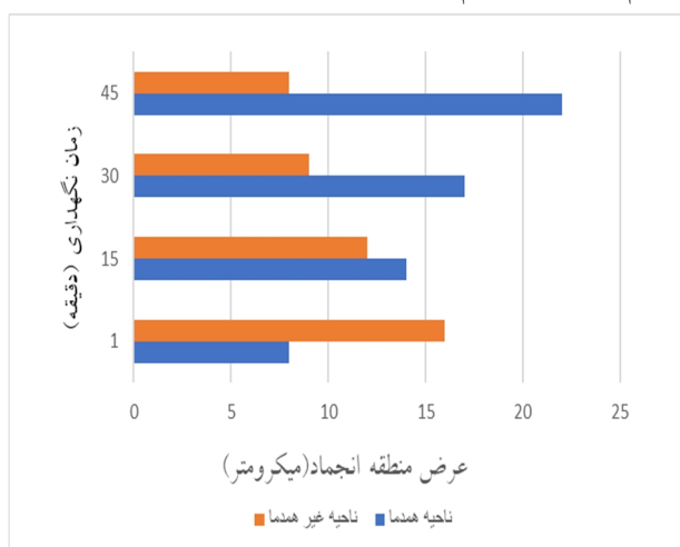
شکل 8- تغییرات عرضی مناطق انجمادی هم دما و غیرهم دما در دمای 1100 درجه سانتی‌گراد و در زمان‌های مختلف.
