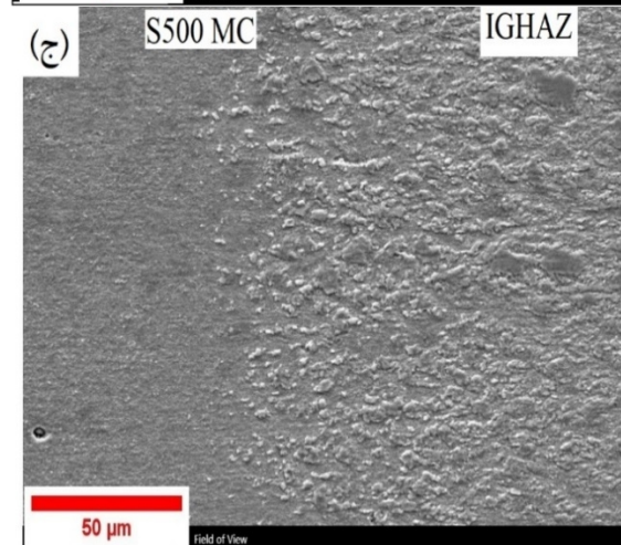
شکل 9- الف- تصویر میکروسکوپ نوری و ب و ج- تصویر میکروسکوپ الکترونی روبشی از نواحی مختلف ناحیه متأثر از حرارت فولاد S500 MC (مقطع TD-ND موقعیت 4 و 5).
