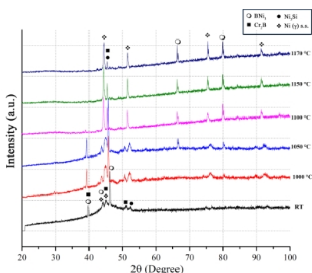
شکل 4- نمودار پراش پرتو ایکس در دماهای مختلف از نیمه مقطع اتصال سمت سوپراآلیاژ.
