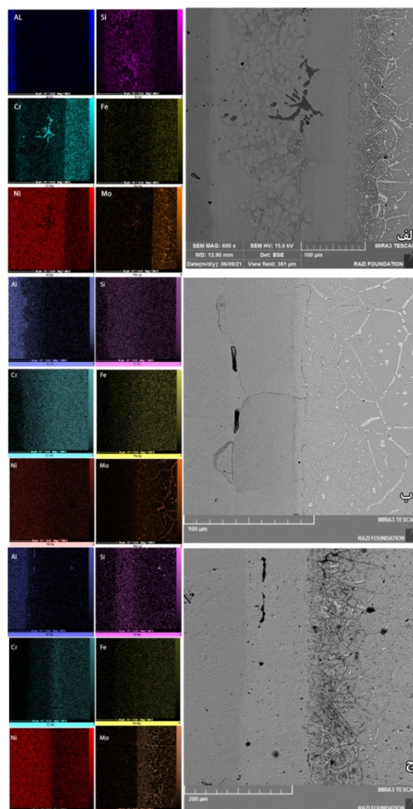
شکل 3- تصویر FESEM به همراه آنالیز MAP نمونه‌های
