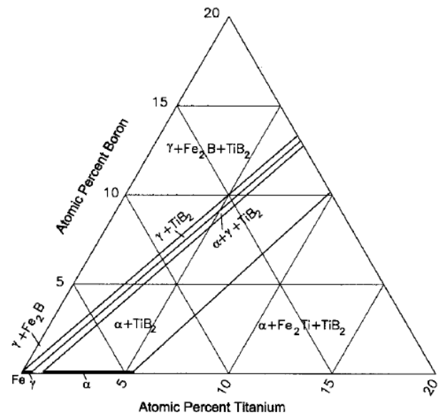
شکل 9- دیاگرام سه‌تایی Fe-Ti-B در دمای 1000^{\circ}\text{C} [27].
