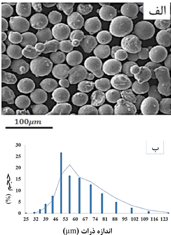
شکل 1- الف - تصویر میکروسکوپی الکترونی رویشی از پودر اینکونل 625 و ب - توزیع اندازه ذرات پودر.
