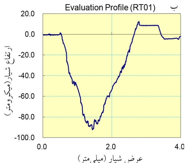
شکل 5- عمق نفوذ و عرض ناحیه سایش یافته زیرلایه و روکش در دمای 25 درجه سانتیگراد.
