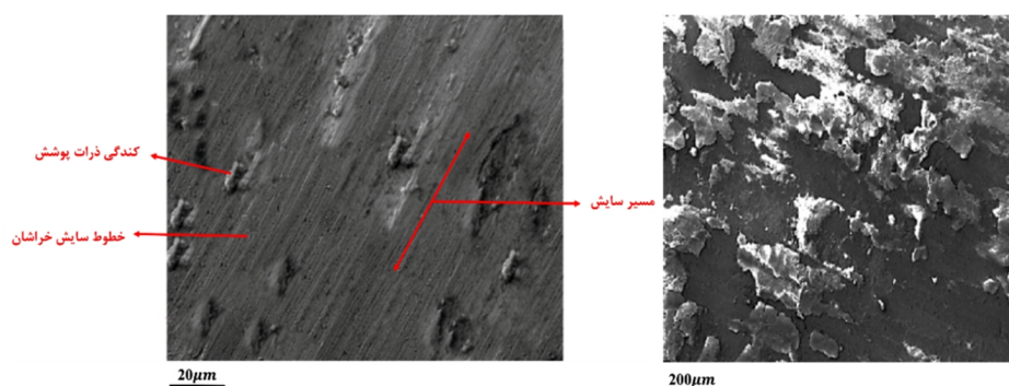
شکل 7- تصویر میکروسکوپی الکترونی روبشی از مسیر سایش زیرلایه در دمای محیط.
