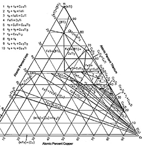
شکل 7- نمودار فازای سه تایی Ti-Fe-Cu.
