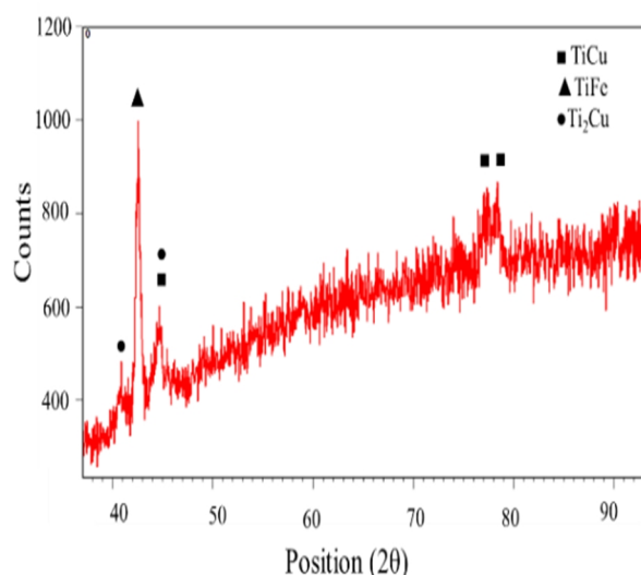
شکل 8- الگوی پراش اشعه ایکس از سطح مقطع اتصال با سرعت جوشکاری 0/9 متر بر دقیقه و میزان انحراف پرتو 0/6 میلی‌متر به سمت تیتانیوم.
