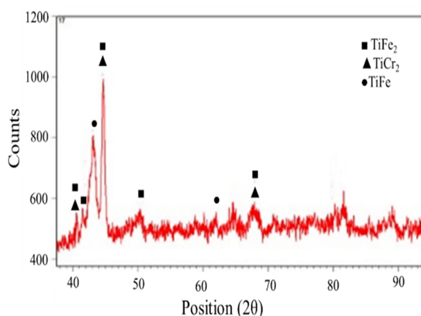
شکل 3- الگوی پراش اشعه ایکس فصل مشترک اتصال مستقیم فولاد 17-4PH به \text{Ti-6Al-4V} .
