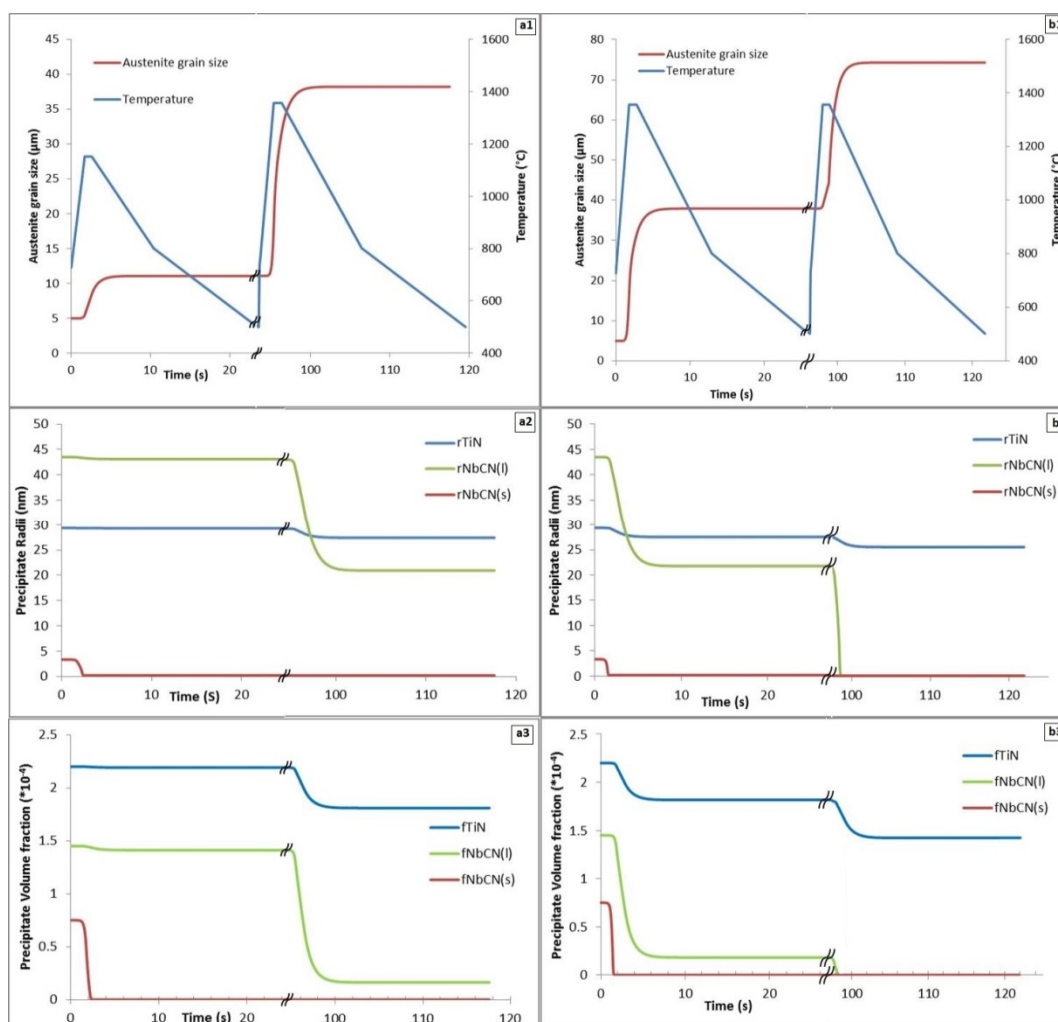
شکل 12-الف- رشد دانه آستنیت پیش بینی شده در چرخه حرارتی نمونه D6 و D9 ب- تغییر شعاع رسوبات و ج- کسر حجمی رسوبات TiN و رسوبات NbC کوچک و بزرگ
