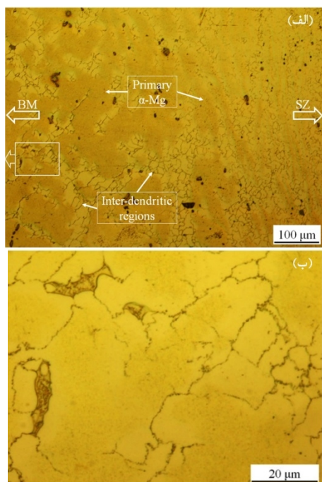
شکل 4- الف - تصویر میکروسکوپ نوری از منطقه ترمومکانیکی نشان دهنده انحلال رسوبات گامای ناپیوسته، فاز \alpha\text{-Mg} اولیه و تبلور مجدد دینامیکی در مناطق بین دندریتی و عدم حضور رسوبات \gamma\text{-Mg}_{17}\text{Al}_{12} یوتکتیک در فواصل نزدیک تر به منطقه همزده شده، ب - تصویر در بزرگنمایی بالاتر از منطقه مشخص شده در الف - نشان دهنده انحلال جزئی و تغییر مورفولوژی داخل رسوبات \gamma\text{-Mg}_{17}\text{Al}_{12} یوتکتیک.
