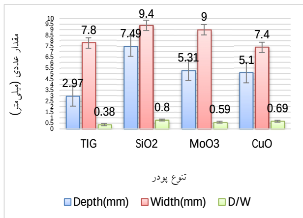
شکل 4- نمودار مقایسه عمق نفوذ، عرض جوش و نسبت عمق به عرض نمونه‌ها.
