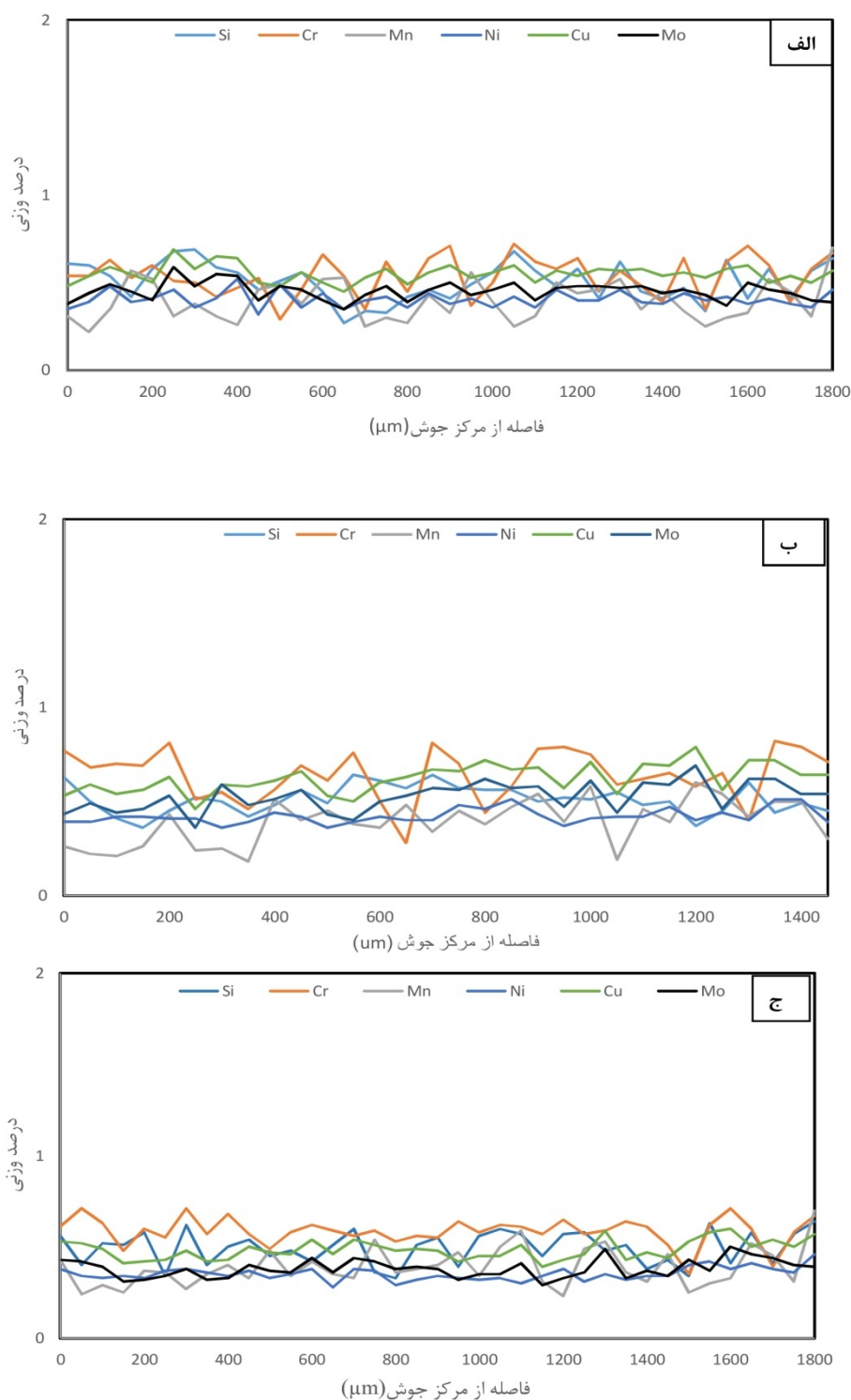
شکل 6- نتایج آنالیز EDS الف - نمونه LW10 ب - نمونه LW11 ج - نمونه LW12.
