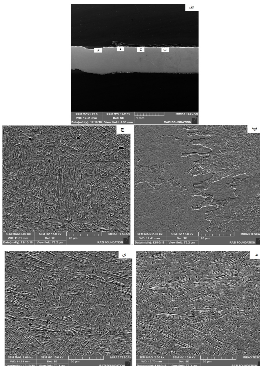
شکل 3- تصاویر میکروسکپی الکترونی، روشی نوای مختلف نمونه LW10
