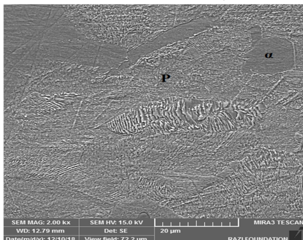
شکل 1- تصویر میکروسکوپی الکترونی روبشی از ریزساختار فولادپایه 1/7225.
