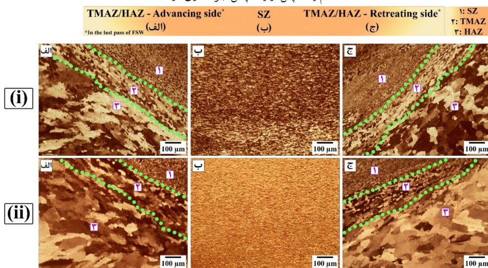
شکل 11- ریزساختار نواحی جوش پس از سه پاس فرایند FSW و در i- \omega/v=25 r/mm و ii- \omega/v=70 r/mm.
