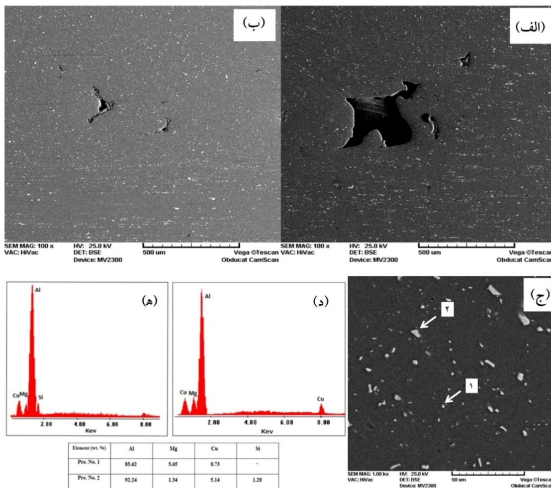
شکل 4- تصاویر میکروسکوپ الکترونی روبشی از منطقه جوش الف- نمونه 11، ب- نمونه 8، ج- رسوبات انتخابی منطقه جوش در تصویر میکروسکوپ الکترونی نمونه 7 جهت آنالیز EDS، د- گراف آنالیز EDS رسوب 1 (نمونه 7) و ه- گراف آنالیز EDS رسوب 2 (نمونه 7).
