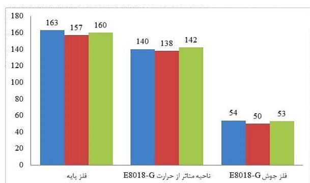
شکل 9- نتایج حاصل از آزمون ضربه شارپی برای نواحی سه گانه حاصل از جوشکاری فولاد P460NH با الکتروود E8018-G.
