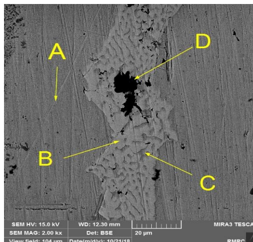
شکل 8 - تصویر میکروسکوپ الکترونی روبشی از محل اتصال نمونه متصل شده در دمای 1120^{\circ}\text{C} و زمان 45 دقیقه. فازهای A, B, C و D در تصویر مشخص هستند که به ترتیب فازهای پرویوتکتیک- \gamma ، بورید غنی از نیکل، یوتکتیک- \gamma و بورید غنی از کروم هستند.
