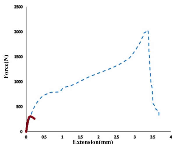
شکل 8- نمودار استحکام کششی قطعات باماده واسطه پلی متیل متاکریلات
