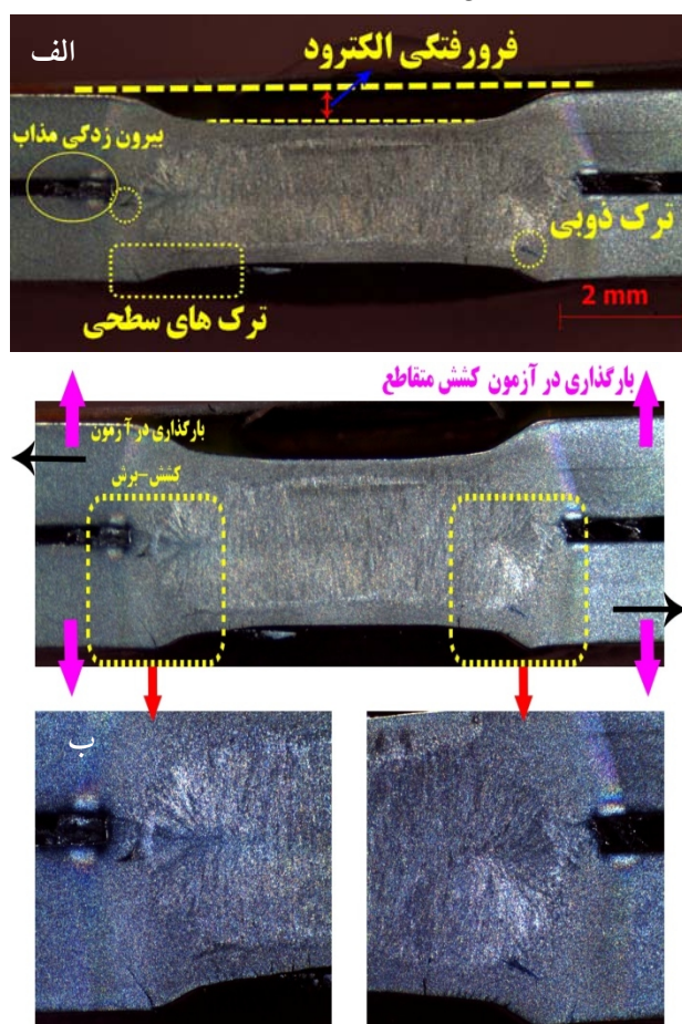
شکل 4-الف) ماکروساختار یک دکه جوش از فولاد TRIP به همراه ع و ناپیوستگی های آن و ب) نحوه بارگذاری های کششی-برشی و کشش- متقاطع به یک جوش حاوی عیوب و ناپیوستگی های جوش.
