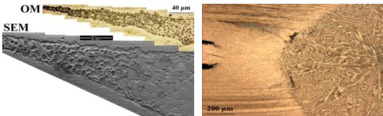
شکل 9- الف) ترک ناشی از روی مذاب، ب) ترک انقباضی و حفره بین دندریتی و ج) ترک ذوبی در جوش های مقاومتی نقطه ای از فولادهای پیشرفته خودروبی.
