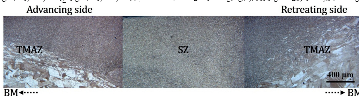
شکل 4- درشت ساختاری از ناحیه اتصال نمونه آنیل شده.
