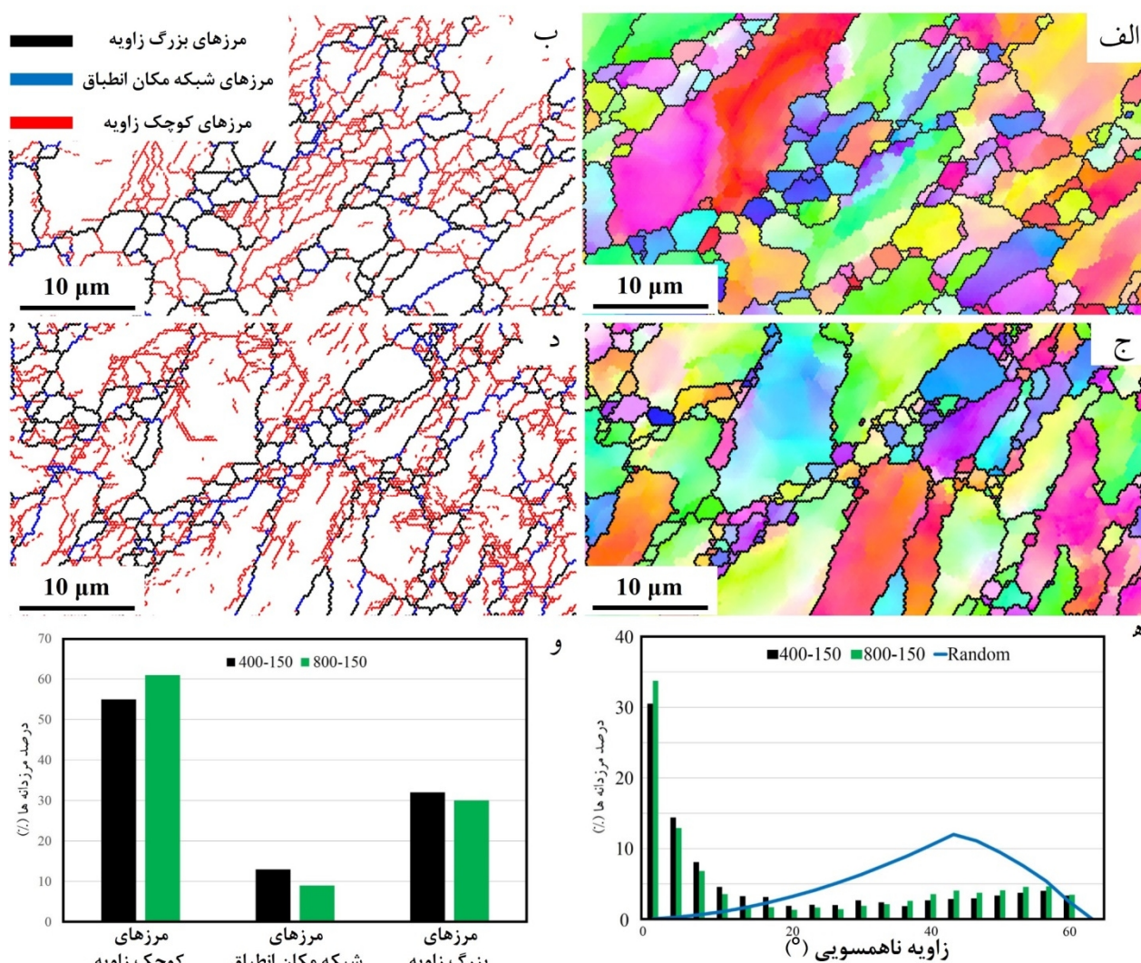
شکل 2- (الف) و (ب) نقشه جهت گیری و مرزدانه ای TMAZ نمونه 400 دور بر دقیقه، (ج) و (د) نقشه جهت گیری و مرزدانه ای TMAZ نمونه 800 دور بر دقیقه، (ه) و (و) منحنی توزیع زوایای ناهمسویی و منحنی درصد نوع مرزدانه ها.
