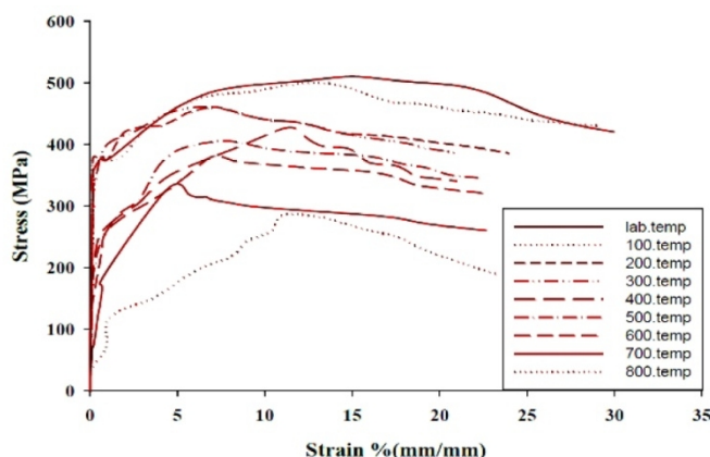
شکل ۲- منحنی های تنش و کرنش تحت دما برای St52 [۲۹]
