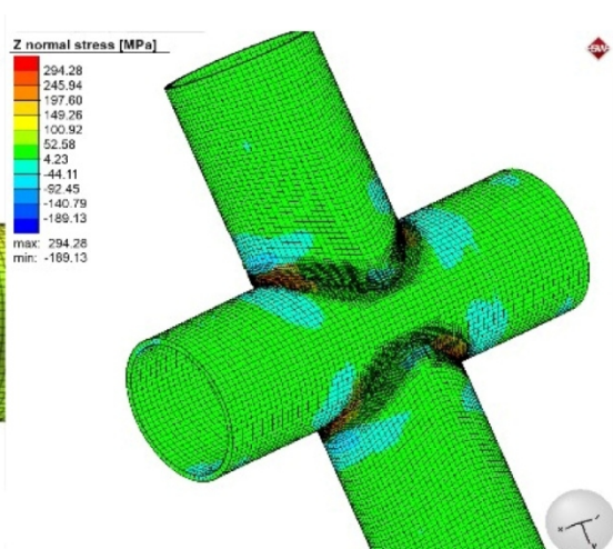
شکل ۱۹- توزیع تنش در راستای Z در اتصال جوشی
