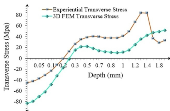
شکل ۲۴- مقایسه نتیجه تنش پسماند عرضی (در راستای محور X) برحسب فاصله از سطح از مدل سازی با نتیجه تجربی
