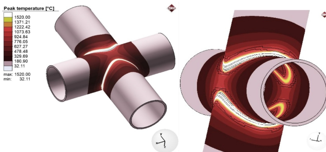
شکل ۱۰- توزیع حرارت در پایان سه پاس جوش که می تواند معیاری برای تخمین ناحیه تحت تأثیر حرارت باشد.
