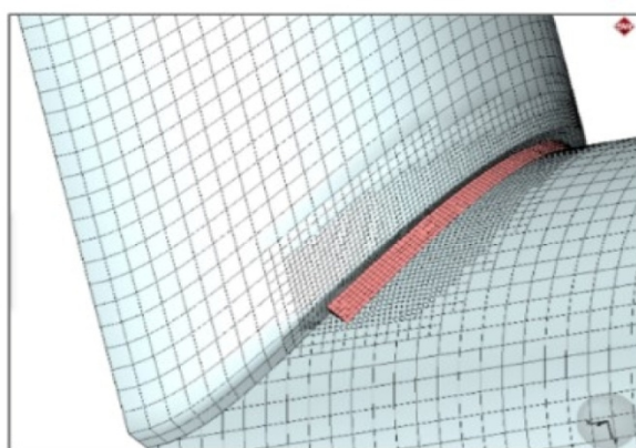
شکل ۵- تکنیک تولد و مرگ المان و اصلاح شبکه بندی با حرکت الکتروود
