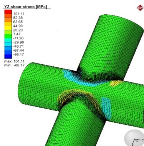
شکل ۲۲- توزیع تنش برشی ( \tau_{yz} ) در اتصال جوشی
