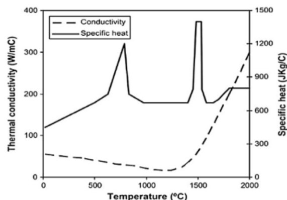
شکل ۱- تغییرات خواص حرارتی St52 با دما [۲۹]
