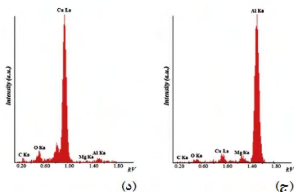
شکل ۱۰- نمونه آنالیز EDS از نقاط ساختارهای لایه ای که با ابزار (الف) و (ب) ساده و (ج) و (د) رزوه ای جوشکاری شده اند
