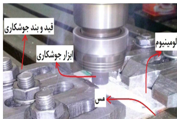
شکل ۱- تصویر فرایند جوشکاری اصطکاکی اغتشاشی
