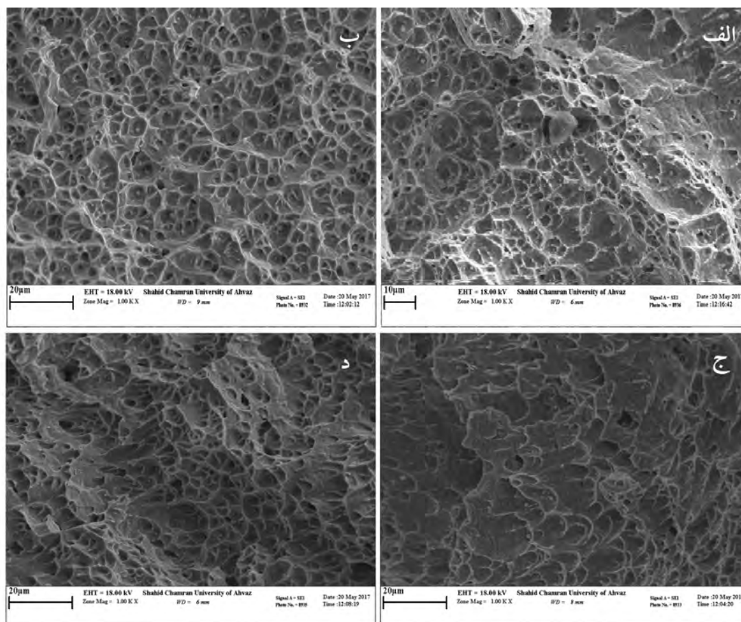
شکل ۸- تصاویر SEM از سطح مقطع شکست فلز جوش ER309L در شرایط مختلف الف- دمای محیط بدون لرزش ب- دمای محیط و لرزش ۳۰ ولت ج- دمای ۲۰۰°C و بدون لرزش د- دمای ۲۰۰°C و لرزش ۳۰ ولت
