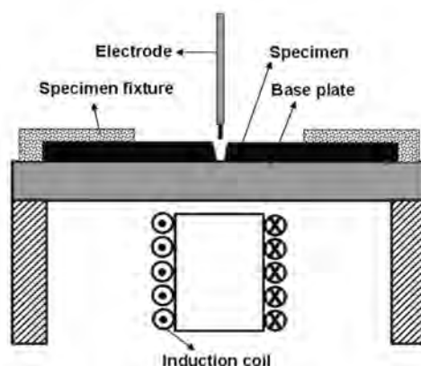
شکل ۱- تصویر شماتیک دستگاه لرزش الکترومغناطیس [۱۶].
