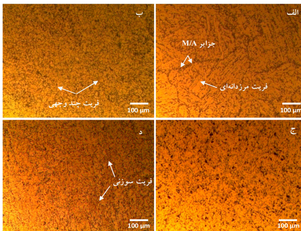
شکل ۳- ریز ساختار فلز جوش ER80S-G در شرایط مختلف الف- بدون لرزش، ب- با لرزش تحت ولتاژ ۲ ولت، ج- با لرزش تحت ولتاژ ۲۰ ولت و د- با لرزش تحت ولتاژ ۳۰ ولت
