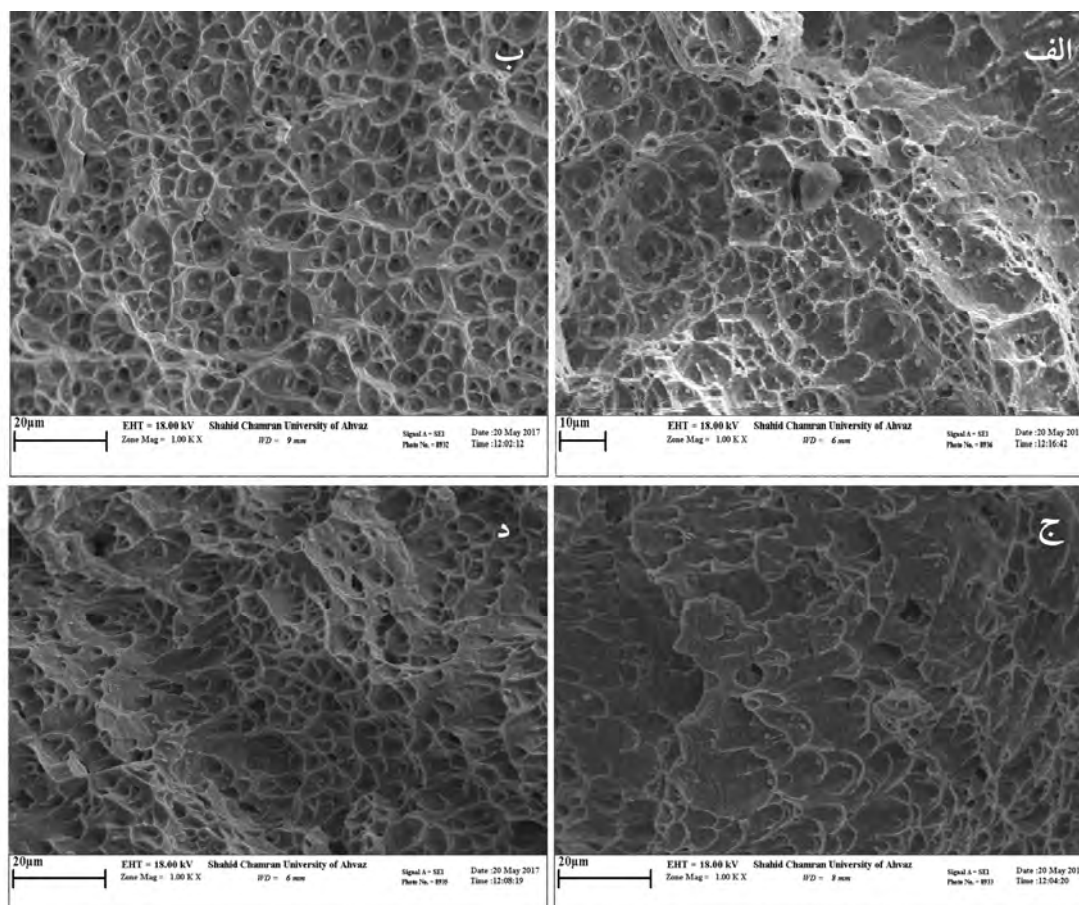
شکل ۸- تصاویر SEM از سطح مقطع شکست فلز جوش ER309L در شرایط مختلف الف- دمای محیط بدون لرزش ب- دمای محیط و لرزش ۳۰ ولت ج- دمای ۲۰°C و بدون لرزش د- دمای ۲۰°C و لرزش ۳۰ ولت
