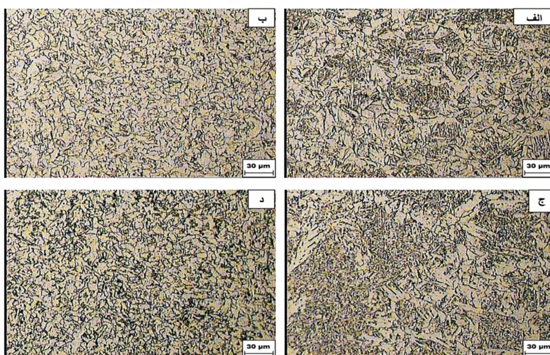
شکل ۷- ریزساختار ناحیه مجدداً گرم شده. (الف و ب) به ترتیب FGRZ و CGRZ مربوط به فلز جوش با ۰ درصد نیکل (ج و د) به ترتیب FGRZ و CGRZ مربوط به فلز جوش با ۱/۲ درصد نیکل
