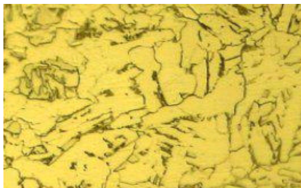
شکل ۱۳- تصاویر میکروسکوپی ناحیه متأثر از حرارت مجاور جوش
