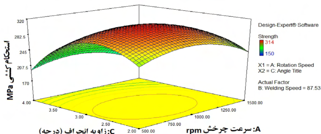
شکل 7- اثر پارامترهای متغیر سرعت دورانی ابزار و زاویه انحراف بر روی استحکام کششی ورق های جوش خورده
