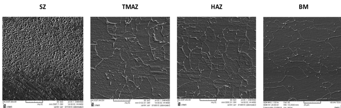
شکل ۱۶- تصویر میکروسکوپ الکترونی نمونه های (a)، مطابق با مناطق مشخص شده در شکل (15)
