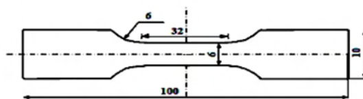
شکل 3- نمونه آزمایش کشش، طبق استاندارد ASTM E8.
