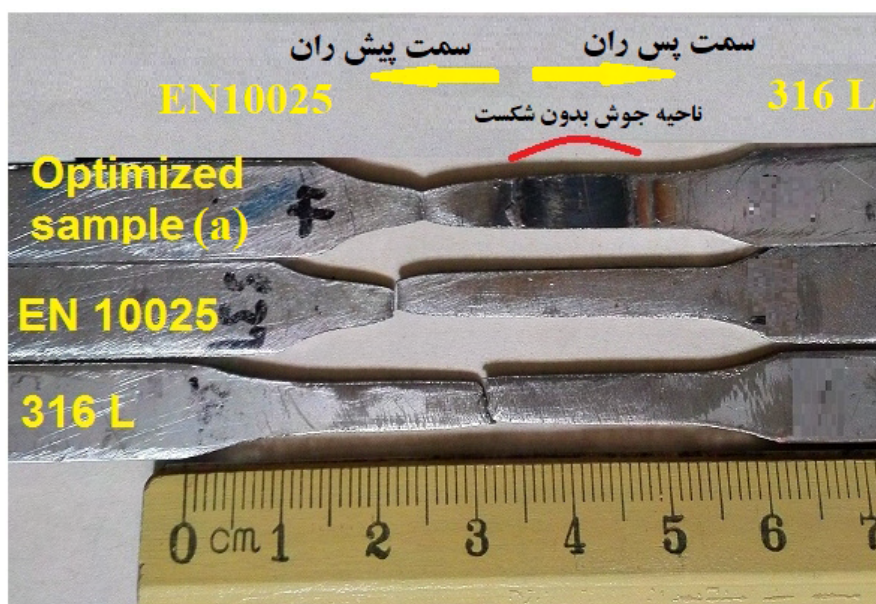
شکل 21- نمونه های آزمایش کشش نمونه بهینه با فلزات پایه.
