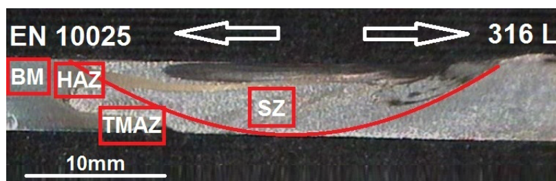
شکل ۱۵- مناطق مشخص شده در تصویر ماکروگرافی و تصویر برداری از مناطق مشخص شده مرتبط با شکل (16).
