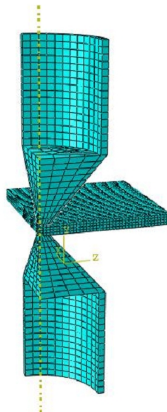
شکل ۷- شبکه بندی مجموعه الکترودها و ورق ها با المان هشت گره ای هگزاهدال Q3D8
