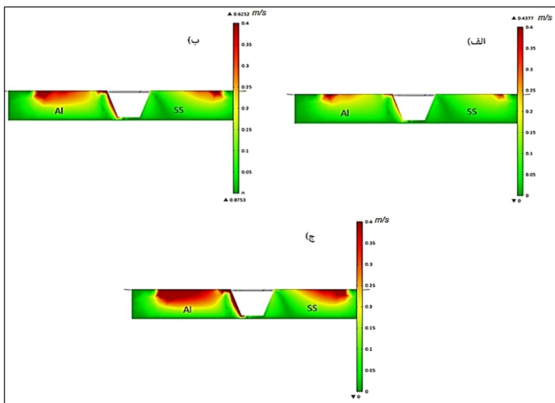
شکل ۱۲- کانتورهای توزیع سرعت سیلان در مقطع درمقطع قطعه در سرعت های چرخشی مختلف. سرعت 350 RPM (الف)، سرعت 500 RPM (ب) و سرعت 700 RPM (ج)
