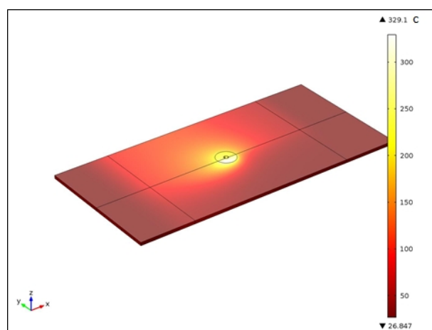
شکل ۹- کانتور توزیع دما شبیه سازی شده در سه بعد
