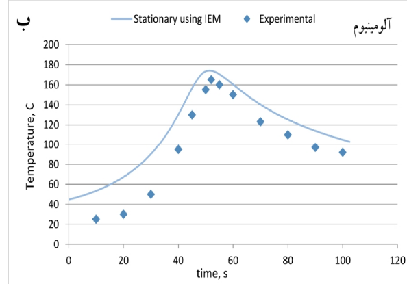
شکل ۸- مقایسه نتایج تاریخچه دمایی برای شبیه سازی و نتایج واقعی در سرعت خطی 80 mm/min
