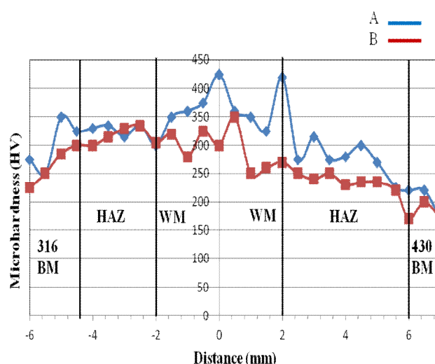
شکل ۱۴- پروفیل سختی از فلز پایه فولاد زنگ نزن فریتی AISI430 تا فلز پایه فولاد زنگ نزن آستنیتی AISI316.
