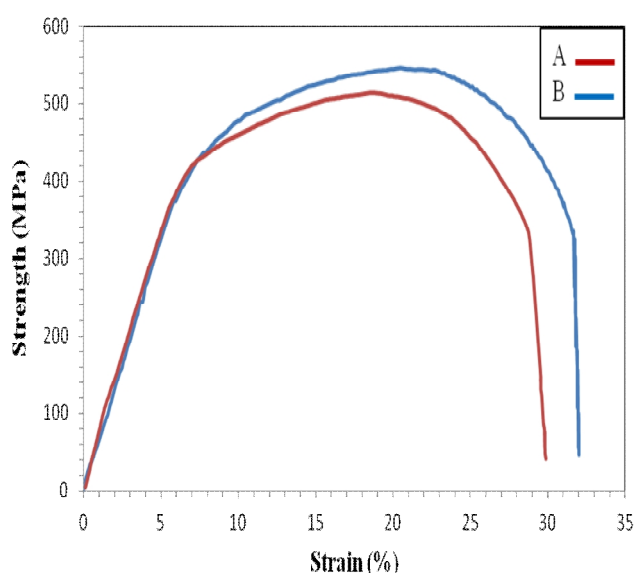
شکل ۱۱- نمودار تنش-کرنش نمونه های جوشکاری شده
